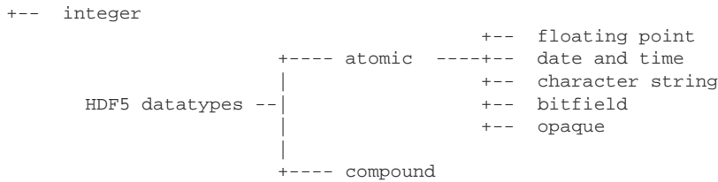
Fig 5.1 HDF5 datatypes
